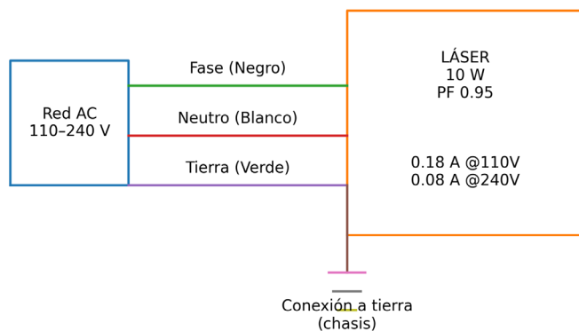
Diagrama de Conexiones Eléctricas
